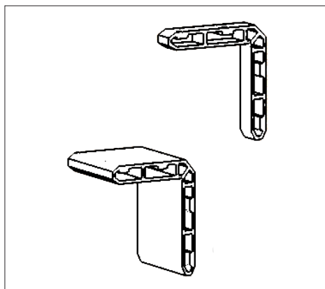
3. Комплект сухарей
